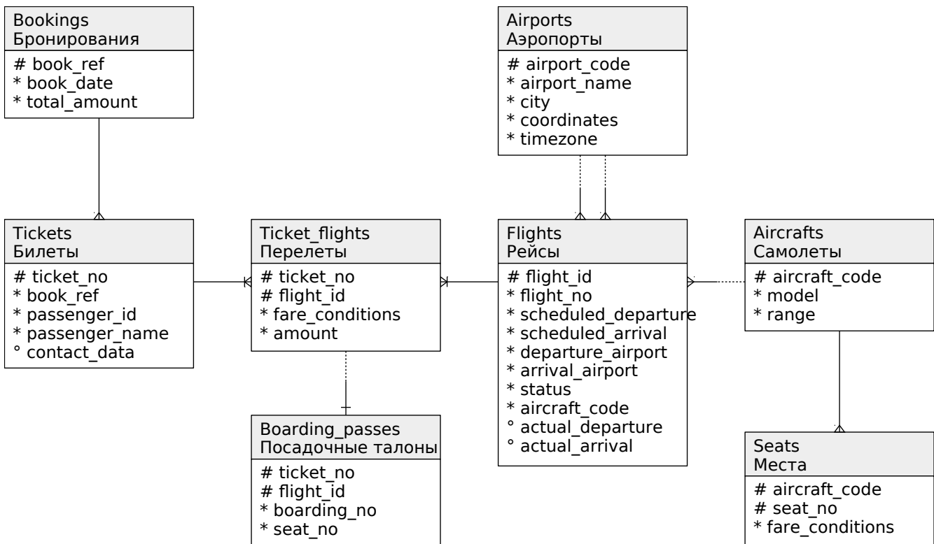
Рисунок К.2. Диаграмма схемы Bookings
