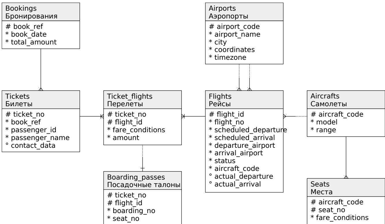
Рисунок М.2. Диаграмма схемы Bookings
